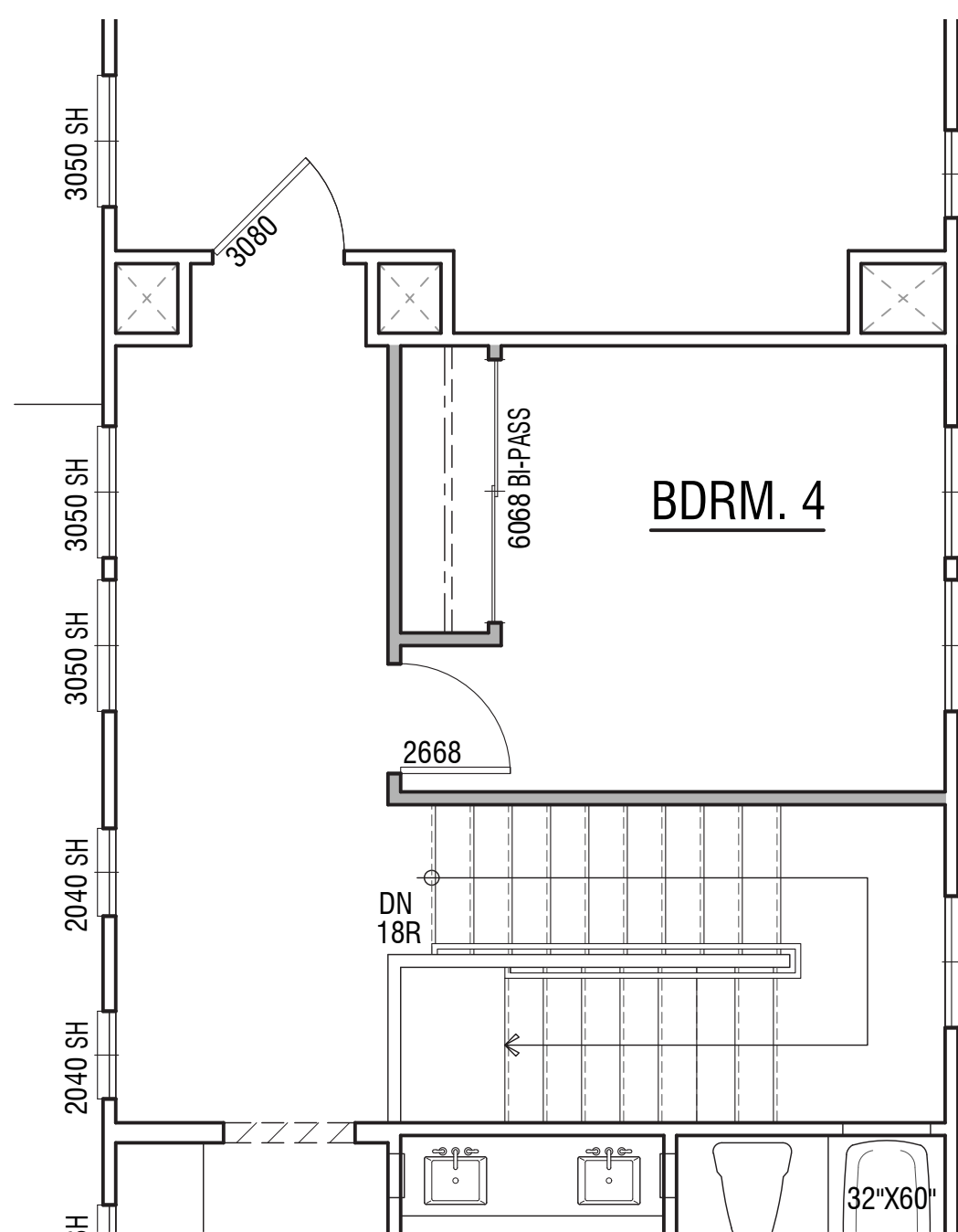
OPTIONAL BDRM. 4 IN LIEU OF LOFT
